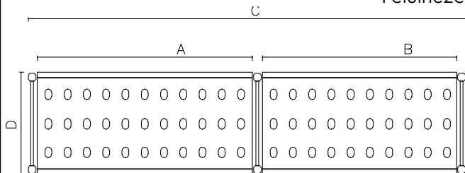
Felülnézet
